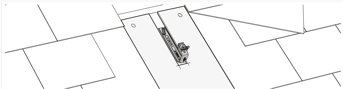
SITUATIE A
