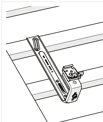
SITUATIE A
