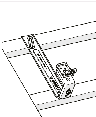
SITUATIE B
